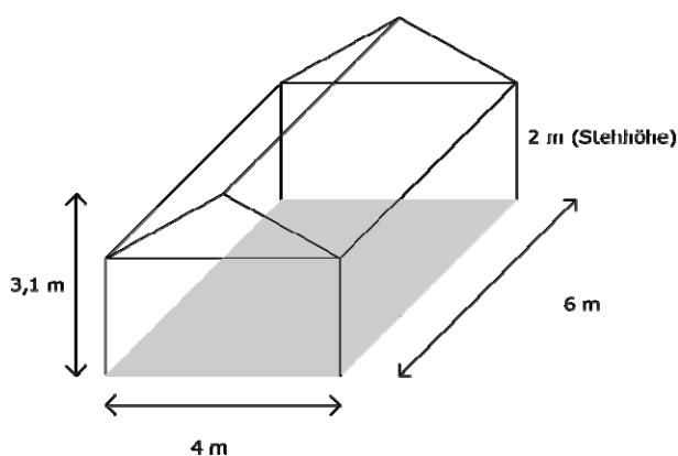
Modell „Satteldach“
